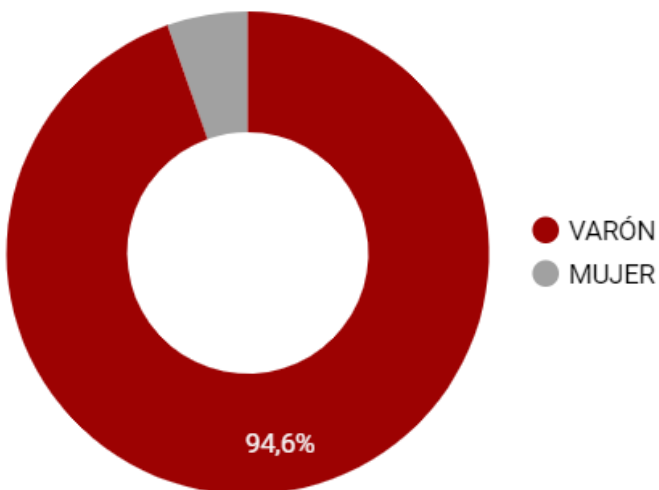
Gráfico N°1: Género
