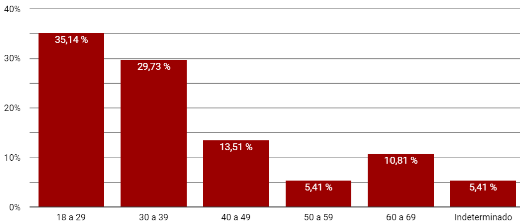
Gráfico N°3: Rango etáreo
